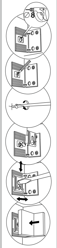
Схема крепления пенала к стене
