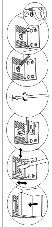
Схема крепления пенала к стене
